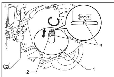
► 1. Plaque de changement 2. Arbre de réglage 3. Flèche
