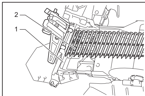
► 1. Glissière de clous 2. Griffes d'alimentation
