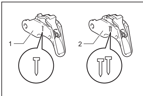
► 1. Gatillo para el accionamiento secuencial simple (color gris) 2. Gatillo para el accionamiento por contacto (color negro)
