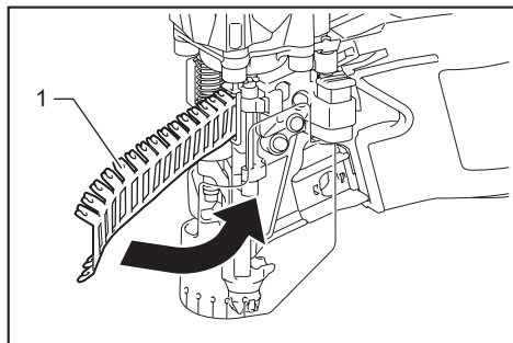
► 1. Lámina intercalada sobresalida
