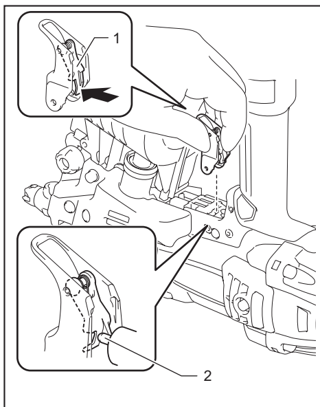
► 1. Parte con bisagra 2. Varilla de la válvula
