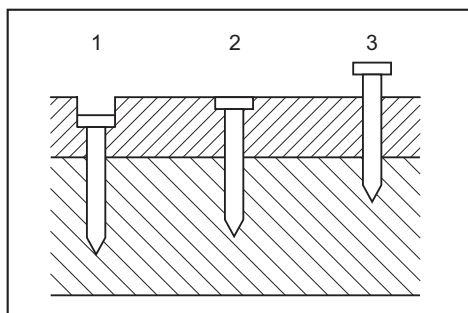
► 1. Trop profond 2. Au même niveau 3. Pas assez profond
