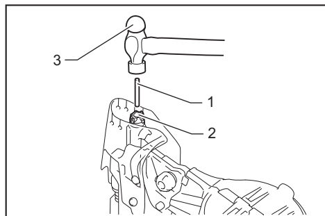
► 1. Tige de métal 2. Sortie d'éjection des clous 3. Marteau
