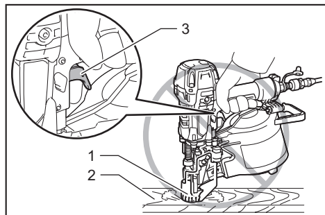
► 1. Elemento de contacto 2. Pieza de trabajo 3. Gatillo (no jalado)
