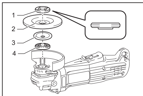
► 1. Contre-écrou 2. Meule flexible 3. Tampon d'ap- point 4. Flange intérieur
