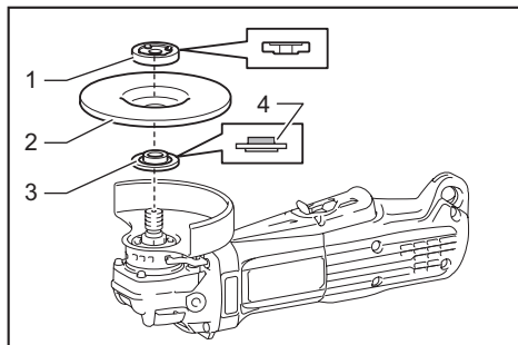
► 1. Contre-écrou 2. Meule à moyeu déporté 3. Flange intérieur 4. Pièce de montage
